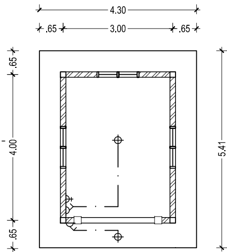
DENAH INSTALASI LISTRIK SKALA 1 : 100
