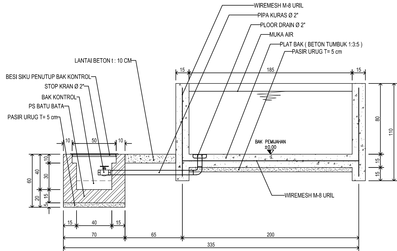
POTONGAN B-B
