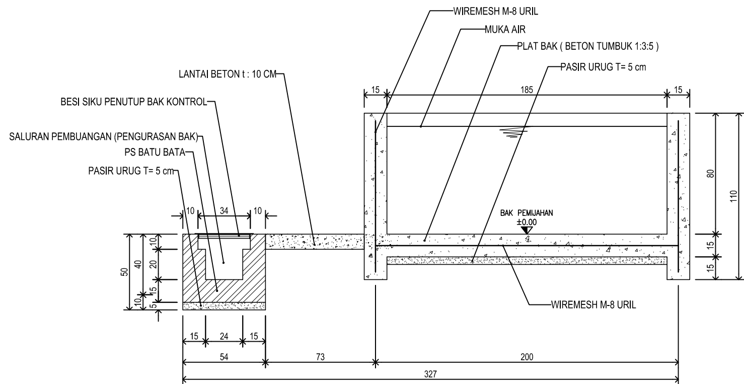
POTONGAN A-A
